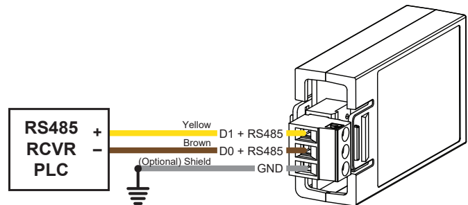
Modbus Module
